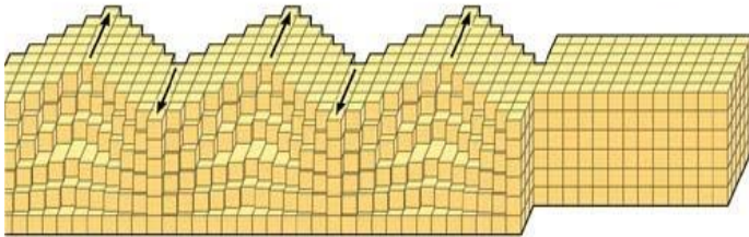
• Love Dalgası
