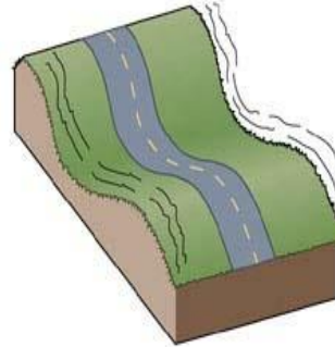
• Rayleigh Dalgası
