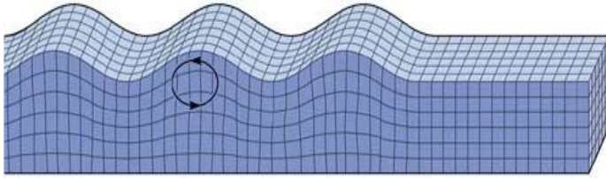
• Rayleigh Dalgası
