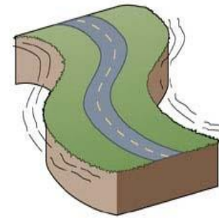
• Love Dalgası
